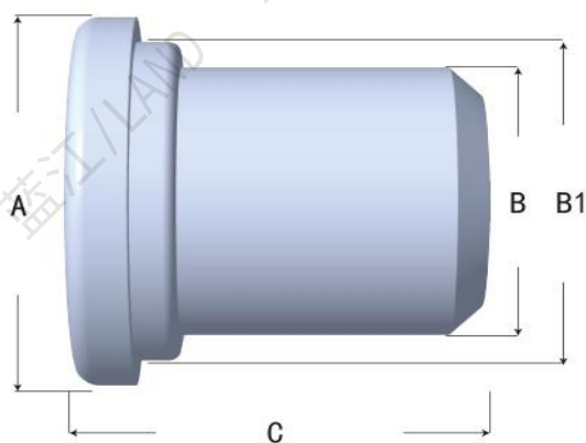
SPR型塞棒
